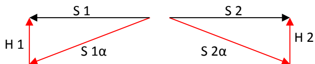
Kräfteplan Aktion
